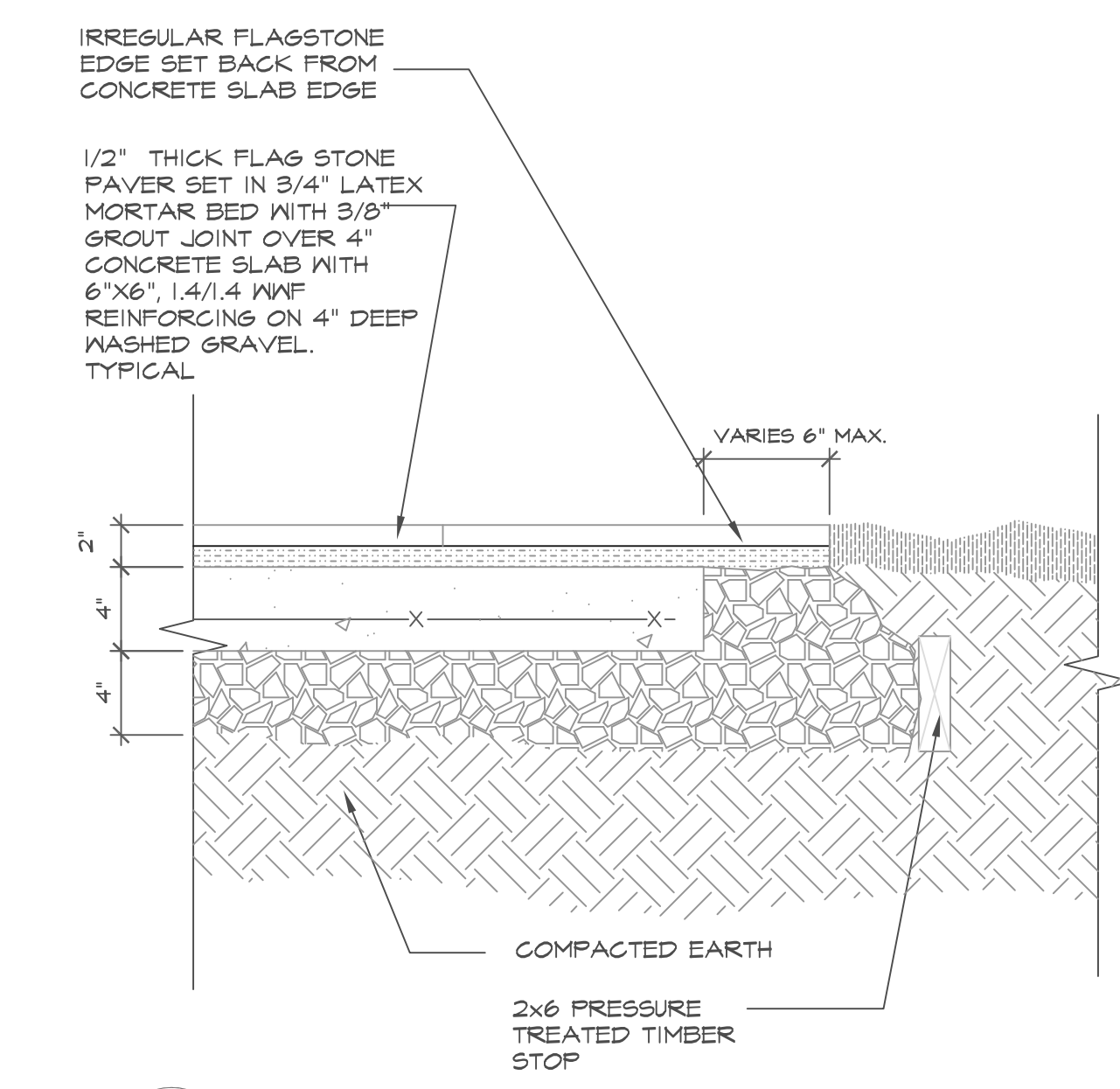
3 STONE EDGE DETAIL SCALE: 1 1/2" = 1'-0"
