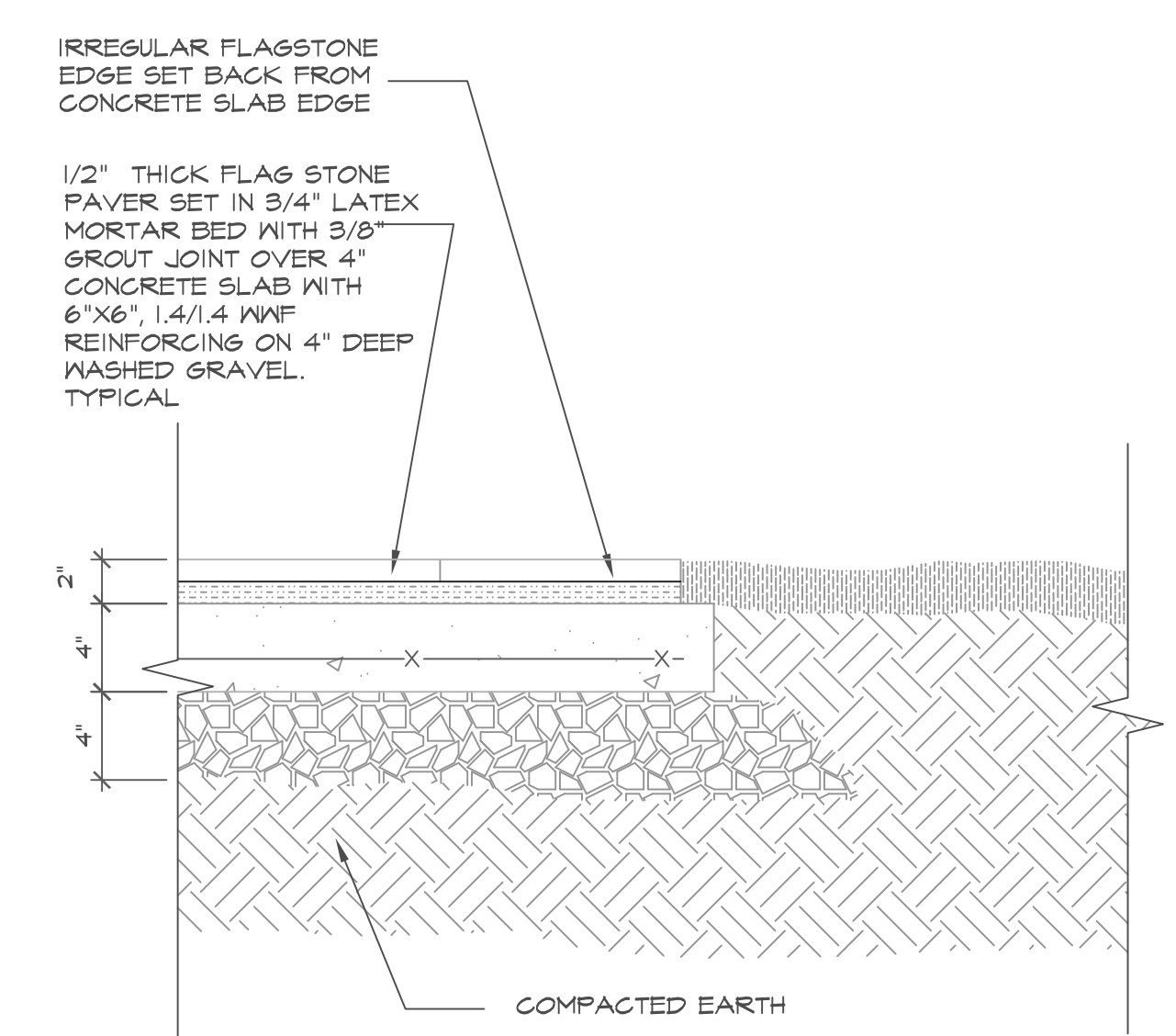
4 ALTERNATE STONE EDGE DETAIL SCALE: 1 1/2" = 1'-0"
